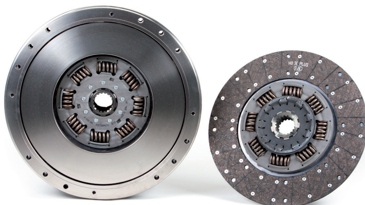
Photo 2 : Embrayage bidisque LuK avec moyeux identiques
