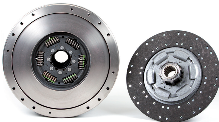
Photo 3 : Embrayage bidisque LuK avec moyeux différents
