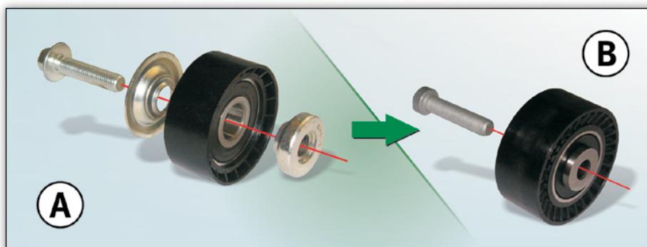
Galet enrouleur 532 0433 10, version précédente (A) et nouvelle version (B)
