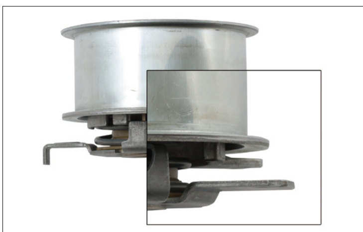
Photo 1 : Etat du galet tendeur à la livraison
