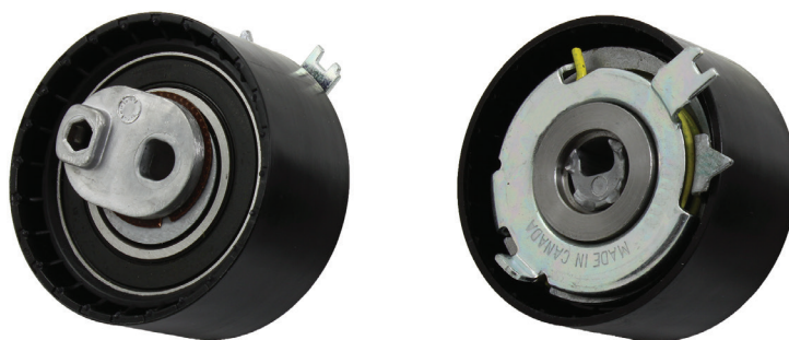
Photo 1 : Galet tendeur INA réf. 531 0710 10
