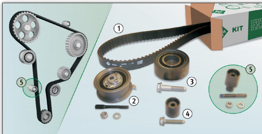
Image 1 : Schéma d'entraînement 1.9 TDI/SDI et contenu du kit 530 0361 10/530 0082 10
