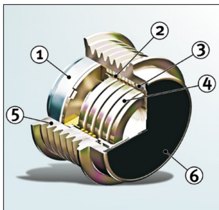
Image 3 : découpleur d'alternateur
