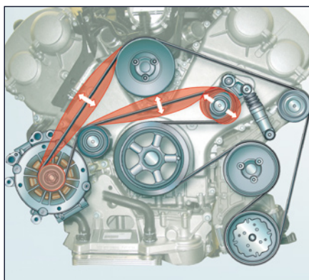
Image 1 : Illustration de l'entraînement des accessoires - dessin des vibrations survenant lors de l'utilisation d'une poulie rigide traditionnelle sur l'alternateur
