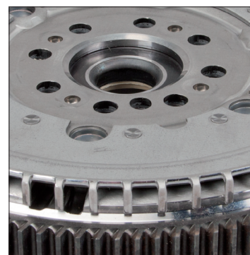
Photo 2: Anneau capteur nouveau modèle
